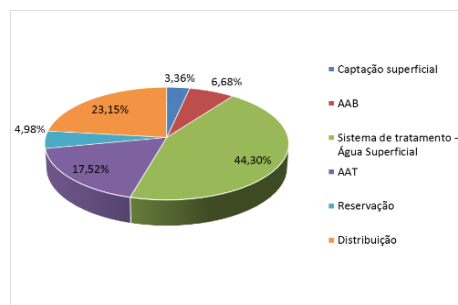
FIGURA 13 – PORCENTAGENS DE INVESTIMENTO PARA O SAA NO DISTRITO DE VERMELHO VELHO - CENÁRIO 2 (FONTE: ELABORADO PELO AUTOR, 2014)
