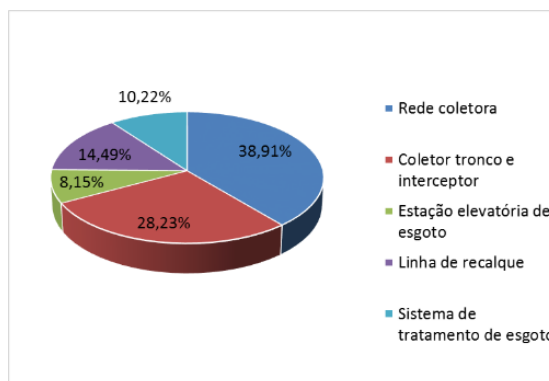
FIGURA 26 – PORCENTAGENS DE INVESTIMENTO PARA O SES NO DISTRITO DE VERMELHO VELHO - CENÁRIO 2 (FONTE: ELABORADO PELO AUTOR, 2014)
