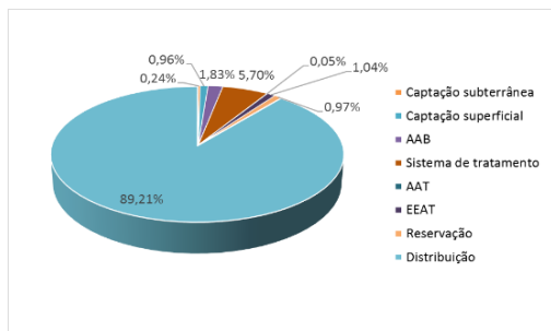
FIGURA 2 – PORCENTAGENS DE INVESTIMENTO PARA O SAA NO DISTRITO SEDE - CENÁRIO 1 (FONTE: ELABORADO PELO AUTOR, 2014)
