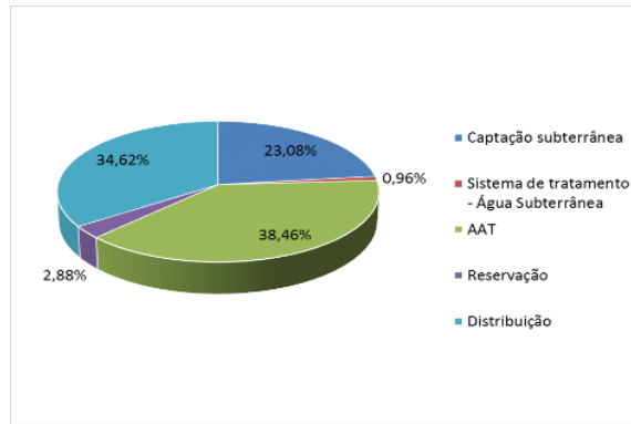
FIGURA 9 – PORCENTAGENS DE INVESTIMENTO PARA O SAA NO DISTRITO DE SÃO SEBASTIÃO DO ÓCULO - CENÁRIO 2 (FONTE: ELABORADO PELO AUTOR, 2014)
