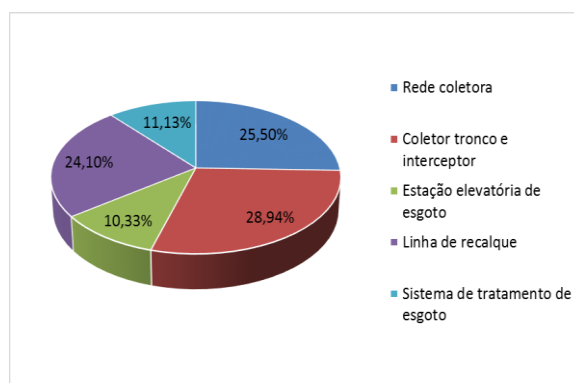
FIGURA 18 – PORCENTAGENS DE INVESTIMENTO PARA O SES NO DISTRITO DE BICUÍBA - CENÁRIO 2 (FONTE: ELABORADO PELO AUTOR, 2014)
