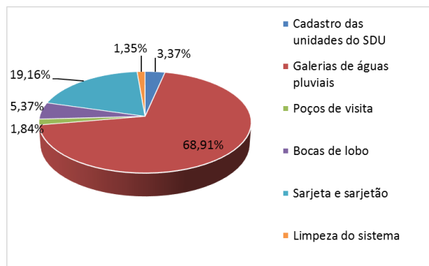
FIGURA 32 - PORCENTAGENS DE INVESTIMENTO PARA SDU NO DISTRITO DE BICUÍBA (FONTE: ELABORADO PELO AUTOR, 2014)
