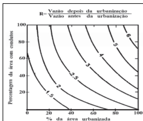
Figura 5 - Aumento do pico em função da proporção de área impermeável e da canalização do sistema de drenagem
