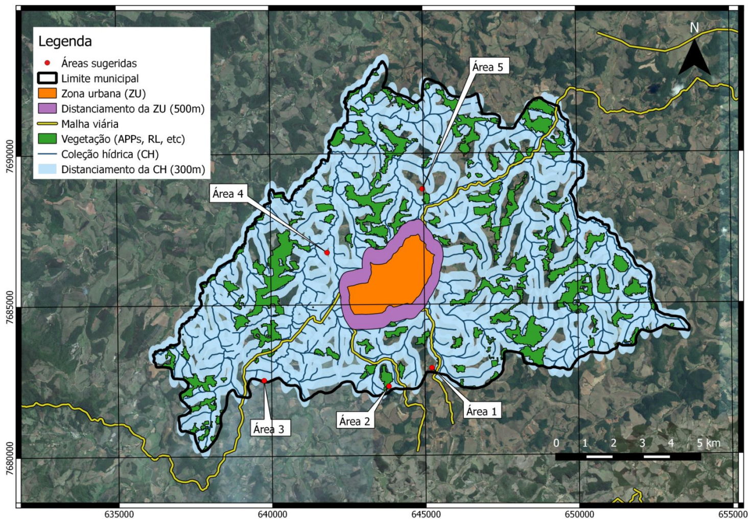
Figura 7 - Áreas sugeridas para instalação do aterro sanitário (AS)
