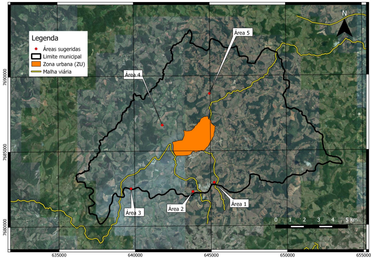
Figura 8 - Áreas sugeridas para instalação do aterro sanitário
