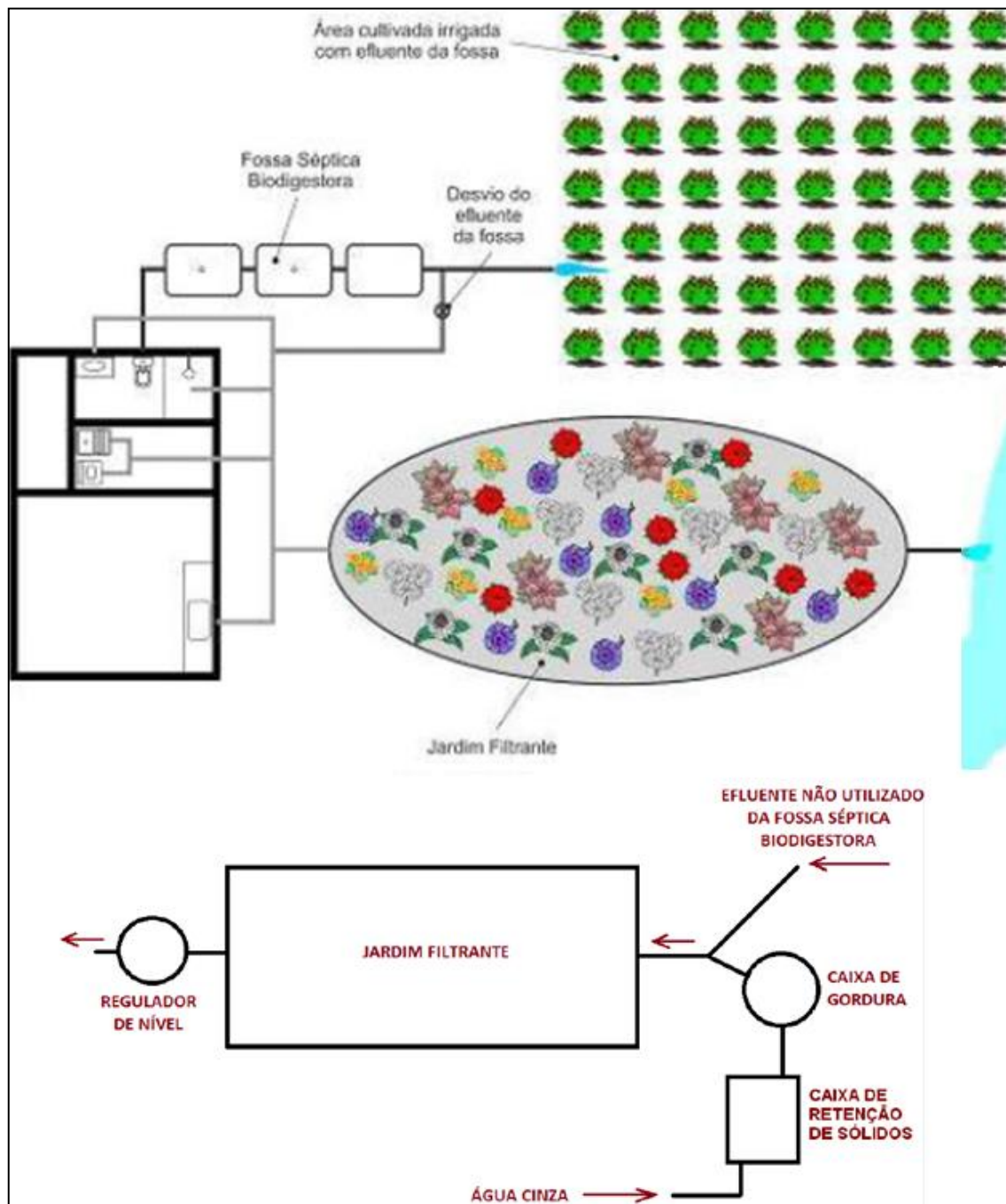
Figura 8 - Ilustração esquemática do Projeto Final
