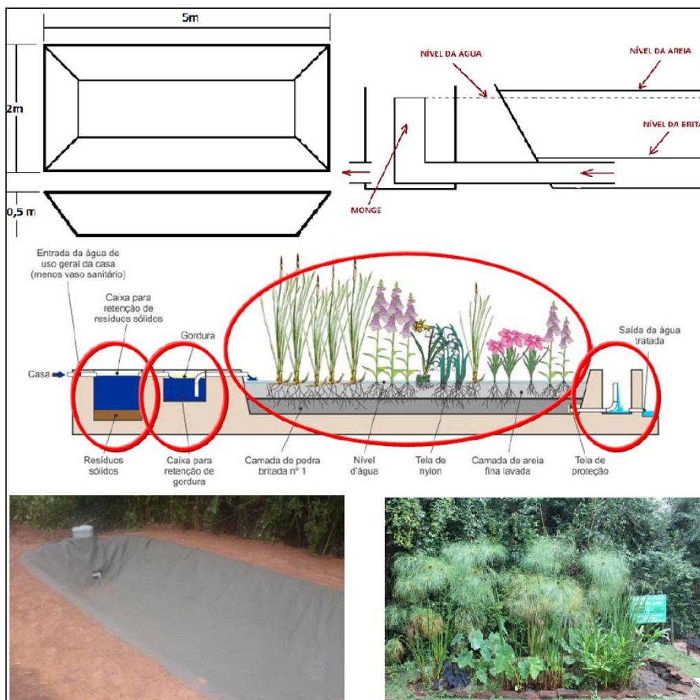
Figura 7 - Ilustração esquemática do Jardim Filtrante desenvolvido pela Embrapa e fotos reais da instalação e projeto finalizado
