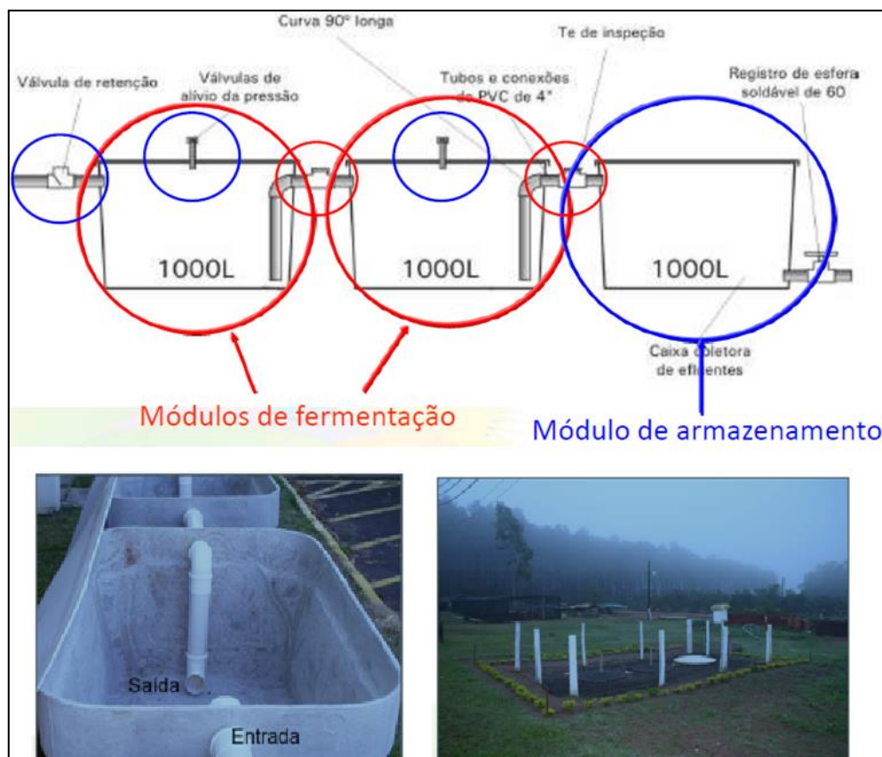
Figura 6 - Ilustração esquemática da fossa biodigestora desenvolvida pela Embrapa e fotos reais da instalação e projeto finalizado
