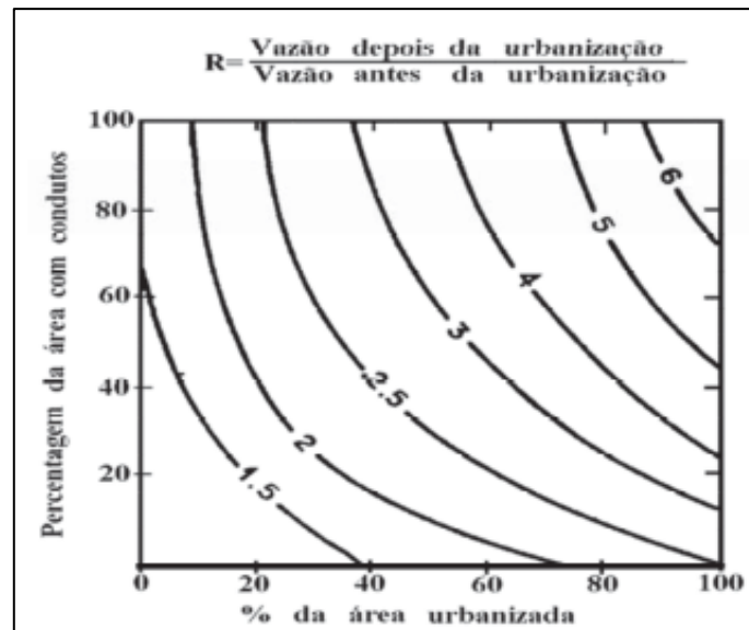
Figura 11 - Aumento do pico em função da proporção de área impermeável e da canalização do sistema de drenagem
