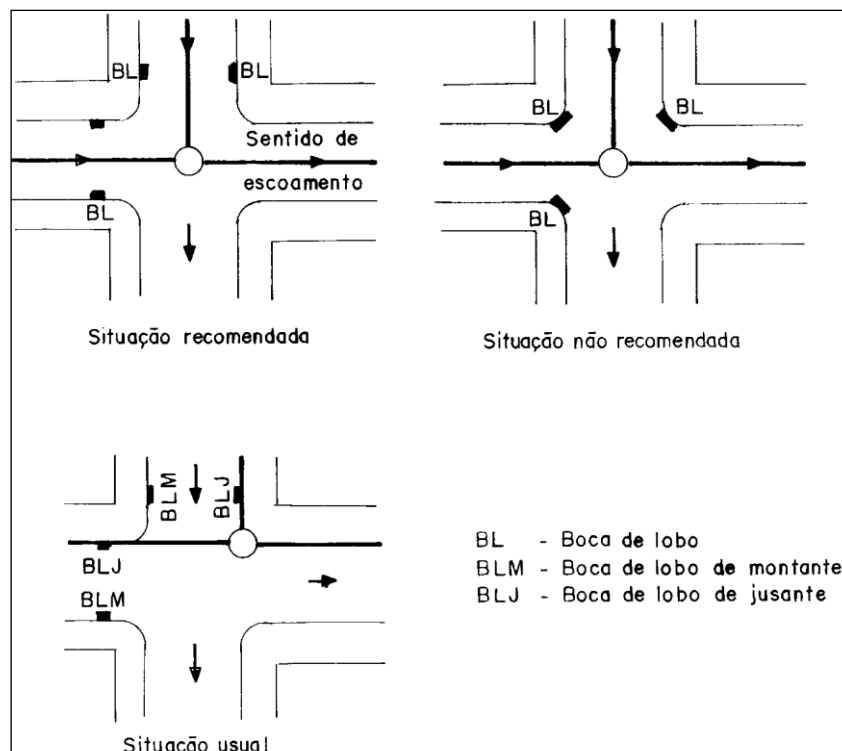
Figura 32 - Rede coletora
