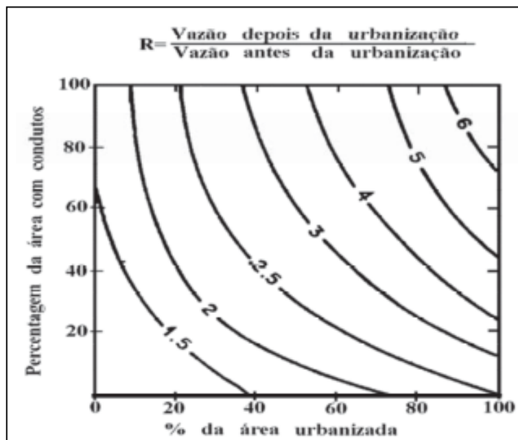
Figura 42 - Aumento do pico em função da proporção de área impermeável e da canalização do sistema de drenagem
