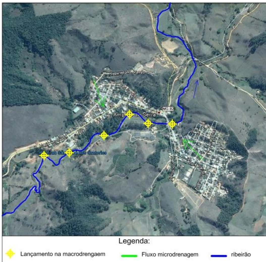
Figura 36 - Croqui dos principais pontos de lançamento da macrodrenagem
