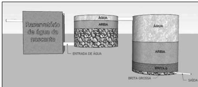
Figura 11 - Esquema geral de filtragem de água de uma nascente
