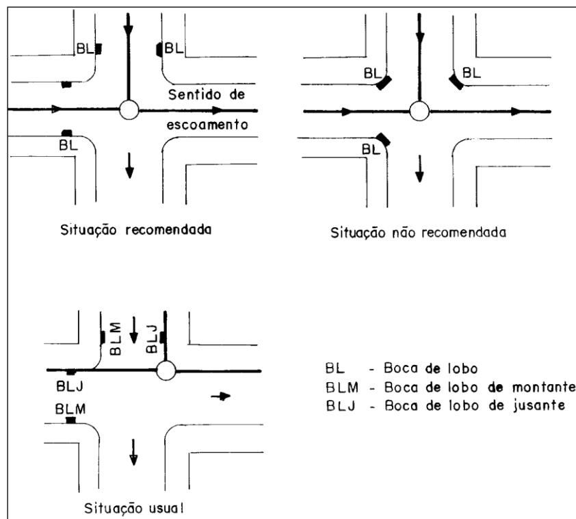
Figura 14 - Rede coletora
