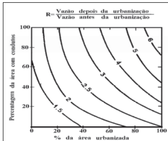
Figura 18 - Aumento do pico em função da proporção de área impermeável e da canalização do sistema de drenagem
