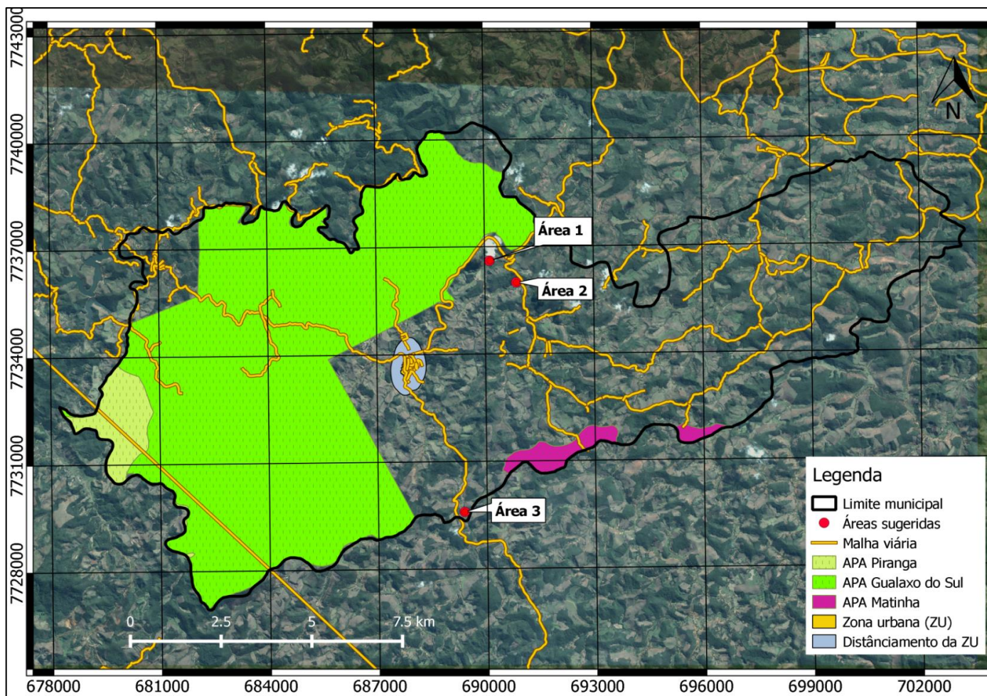
Figura 26 - Áreas sugeridas para instalação do aterro sanitário (sem APPs)
