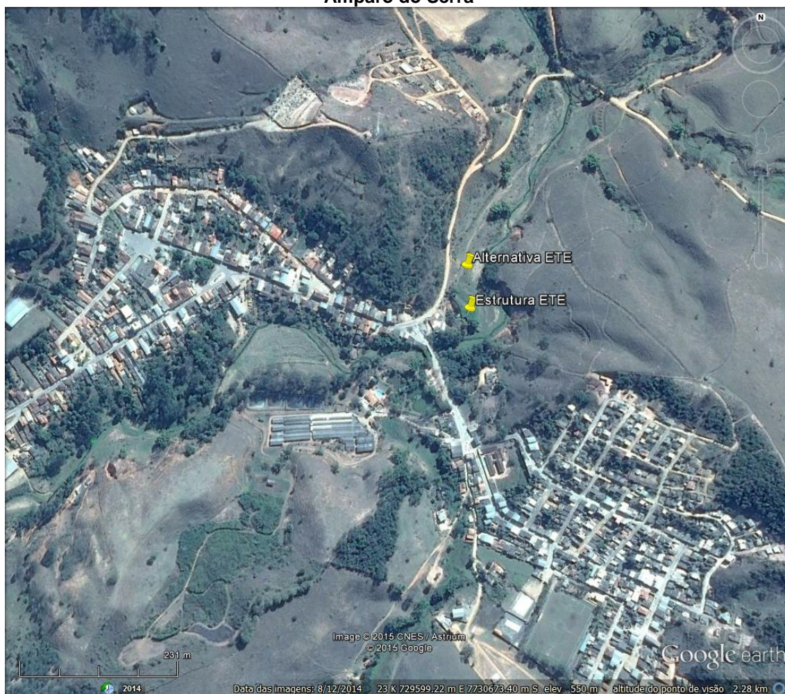
Figura 3 - Alternativa locacional para a instalação de uma ETE na sede do município de Amparo do Serra
