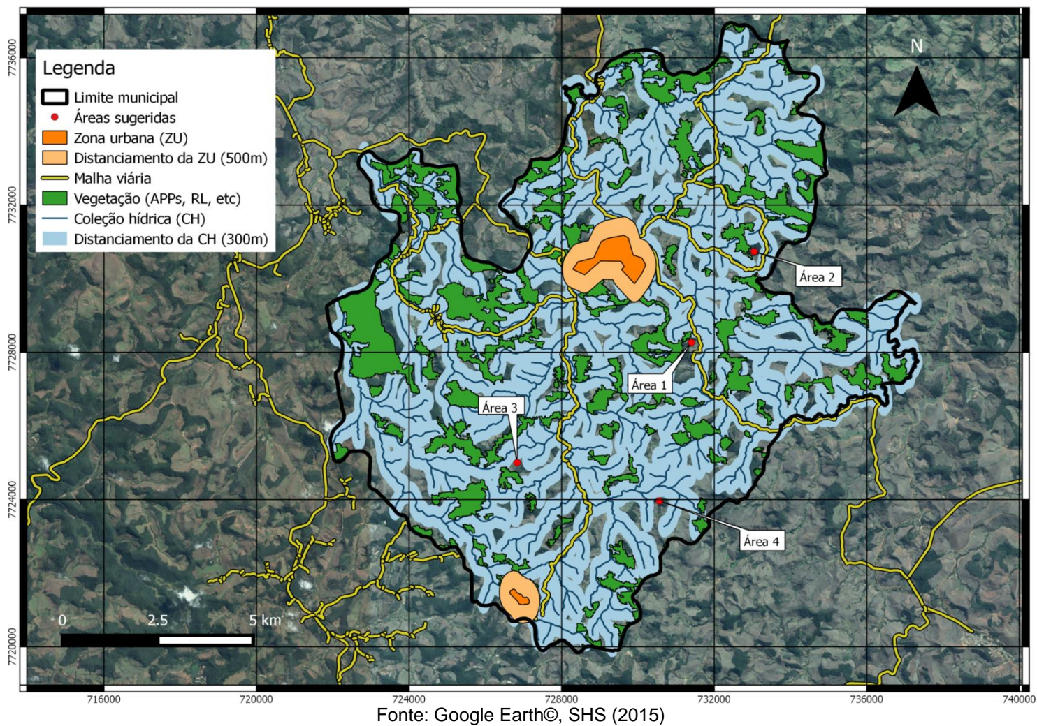
Figura 5 - Áreas sugeridas para instalação do aterro sanitário (AS), em Amparo do Serra - MG
