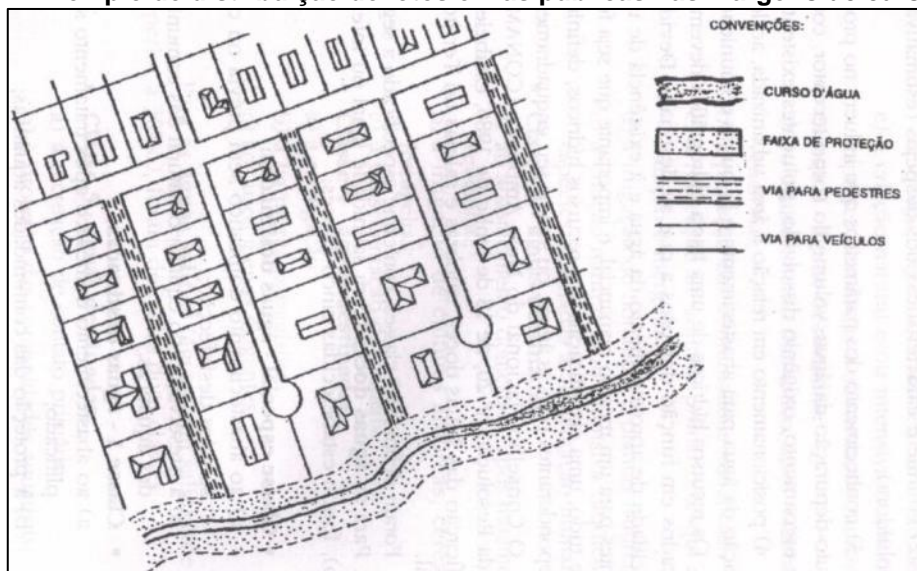
Figura 82 - Exemplo de distribuição de lotes e vias públicas nas margens de cursos d'água
