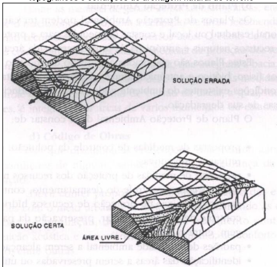
Figura 83 - Exemplo de parcelamento do solo considerando aspectos topográficos e condições de drenagem natural do terreno
