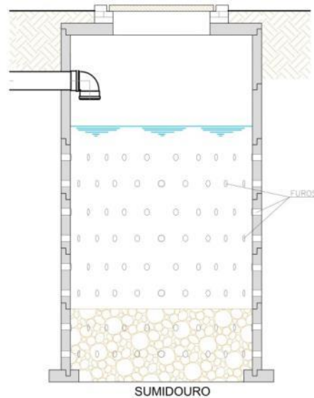
Figura 76 - Esquema de um sumidouro
