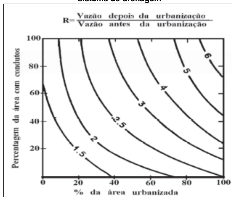
Figura 78 - Aumento do pico em função da proporção de área impermeável e da canalização do sistema de drenagem
