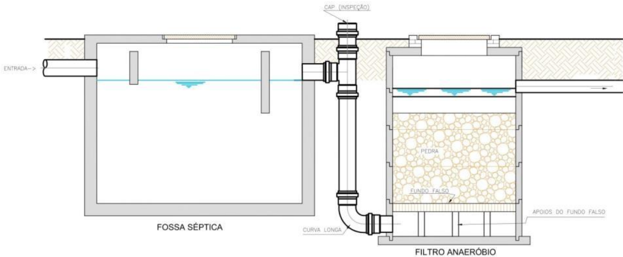
Figura 75 - Esquema do sistema de fossas/tanques sépticos em conjunto com o filtro anaeróbio
