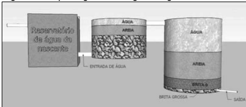
Figura 73 - Esquema geral de filtração de água de uma nascente
