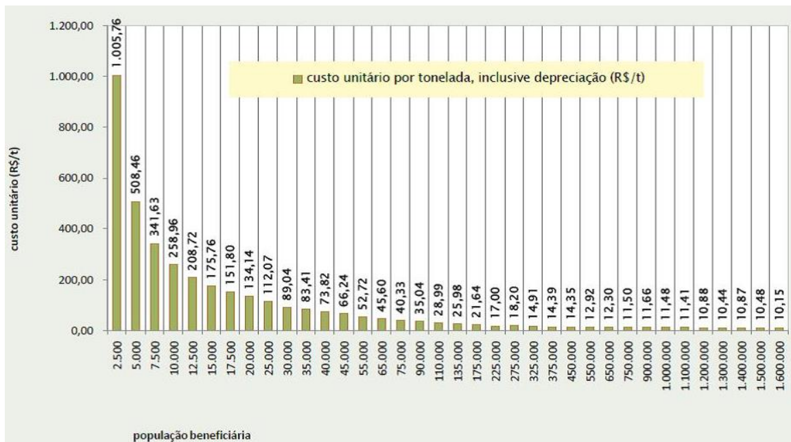
FIGURA 15 – CUSTO ESTIMADO DE OPERAÇÃO DE ATERRO SANITÁRIO (FONTE: VELLOSO, 2010 APUD TCU, 2011)
